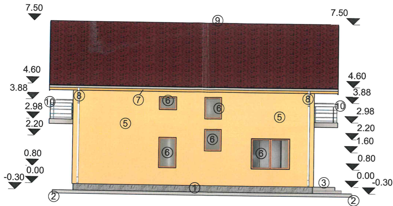
FATADA POSTERIOARA
