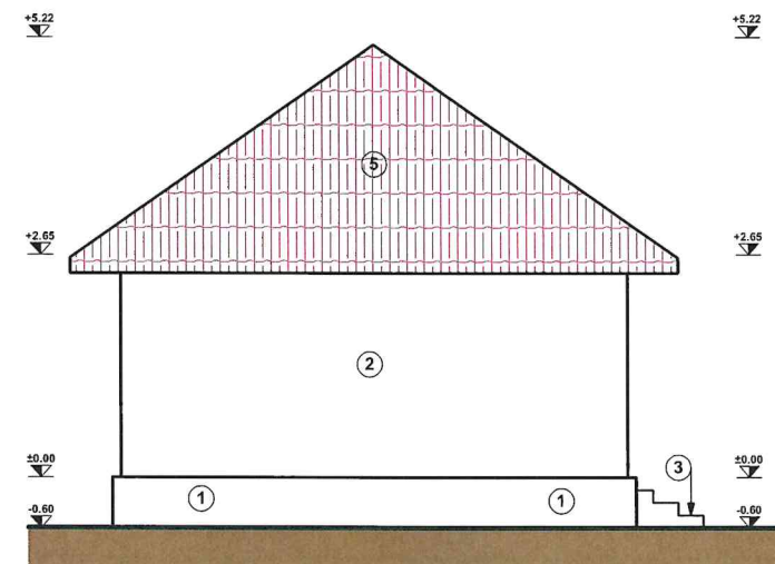
Fatada casa de locuit P - C1 Fatada nord-est
